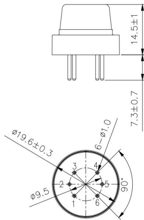
图 1 传感结构图
