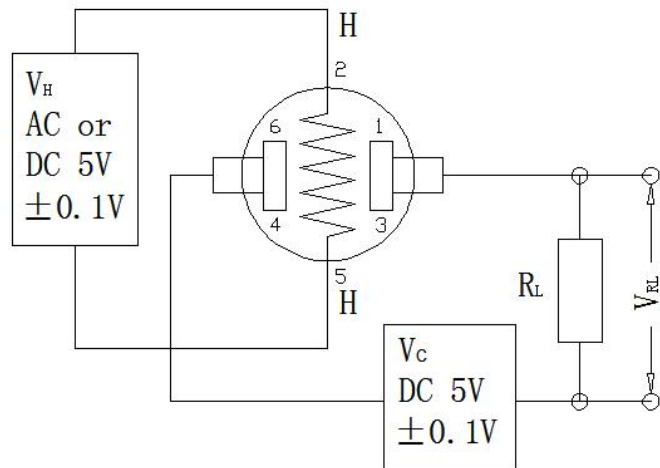
图 2 测试电路
